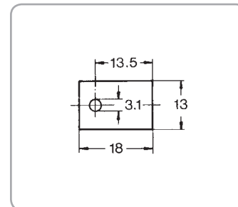
Art.-Nr.: KU 6-623 TO-220
