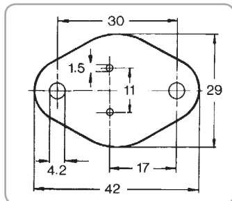
Art.-Nr.: KU 6-619 TO-3
