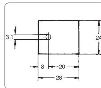
Art.-Nr.: KU 6-630 TO-3PL · TO-264
