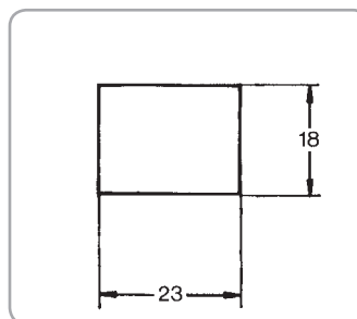
Art.-Nr.: KU 6-628/0 TO-220
