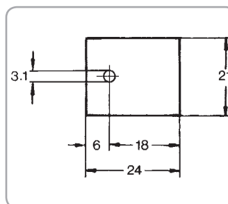
Art.-Nr.: KU 6-624 TO-3P · TO-218/247/248 · MT 100
