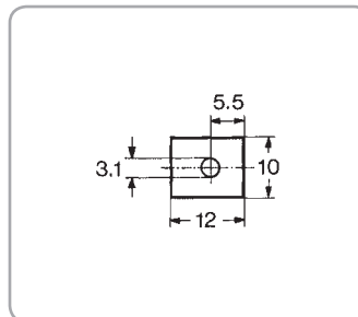
Art.-Nr.: KU 6-620 TO-126 · SOT-32
