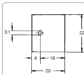
Art.-Nr.: KU 6-631 Multiwatt
