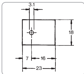
Art.-Nr.: KU 6-628 TO-220
